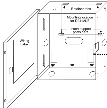
Figure 2: D2803 Enclosure
